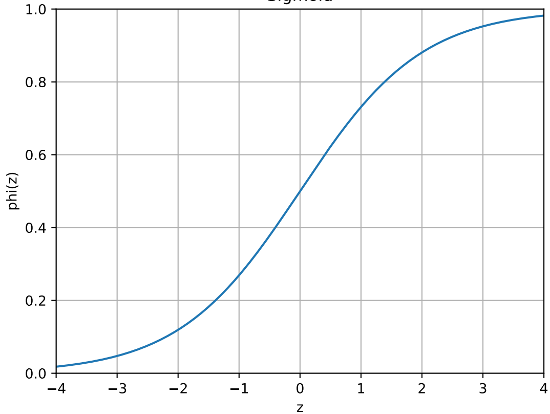
Sigmoid
